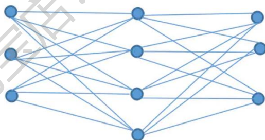
10顶点边数最多三部图模型
