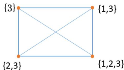
R的第二种关系图
