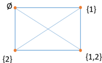
R的第一种关系图
